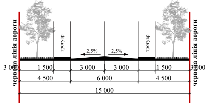
Розріз II-II по вул. Біласа і Данилишина М 1:200
