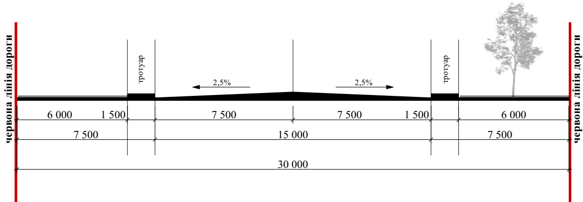
Розріз I-I по вул. Ринкова М 1:200
